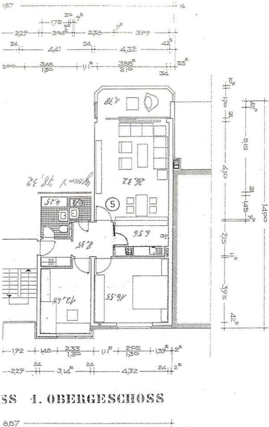
Grundrissplan
